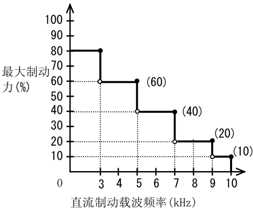
直流制动力限制 (75kW~132kW)
