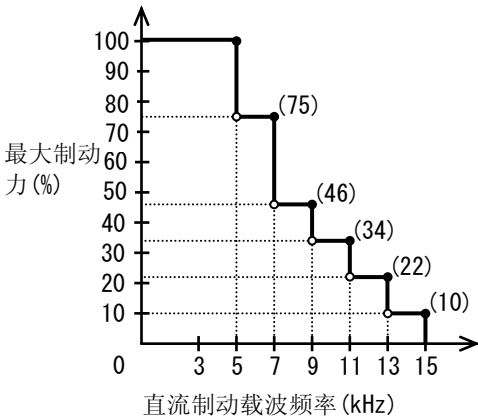
直流制动力限制 (~55kW 以下)
