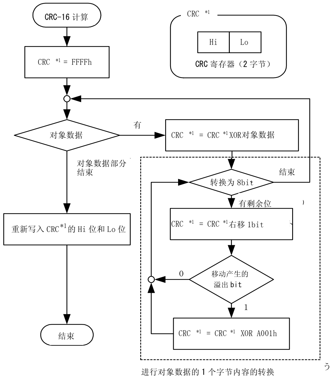
CRC-16 计算步骤例
