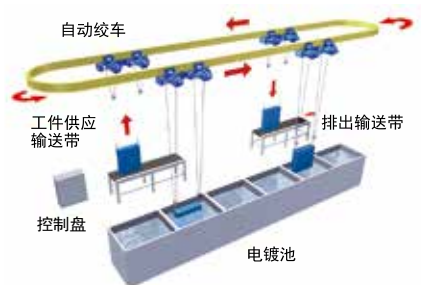
自动输送绞车系统
