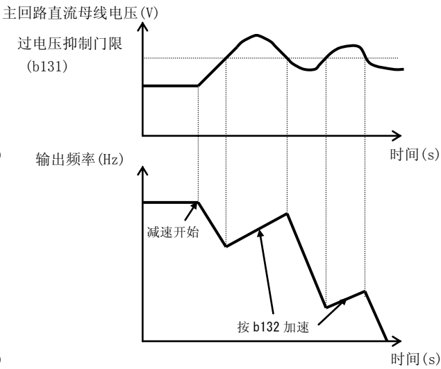
例 2) 设定 b130=02 时
