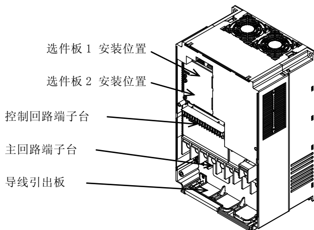
取下表面盖板・端子台盖板后的状态
