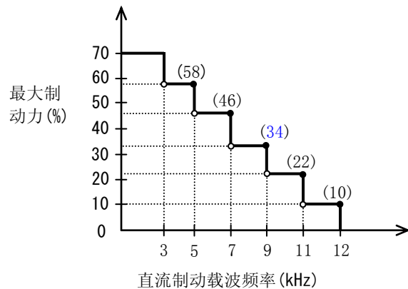
直流制动力限制 (5.5~75kW)
