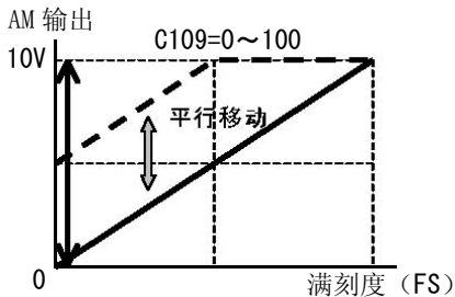
AM 偏置调整
