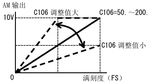
AM 增益调整
