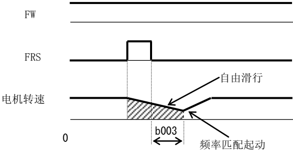
(例2) 频率匹配起动
