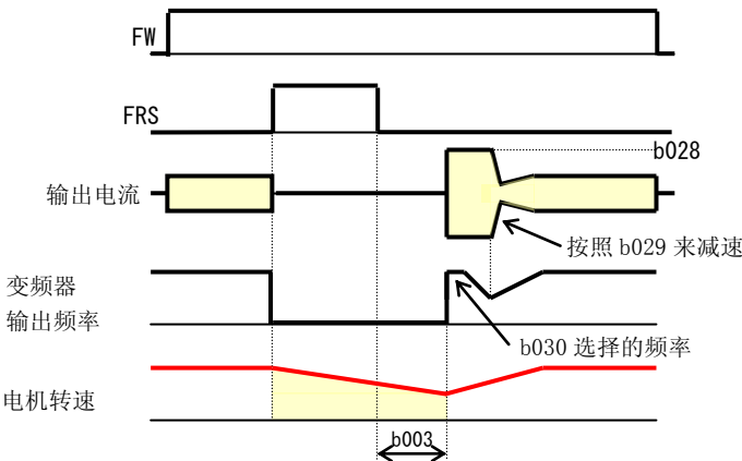
(例 3) 频率引入重起动
