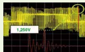
变频器直流母线电压: 625V 电缆长度: 100m
