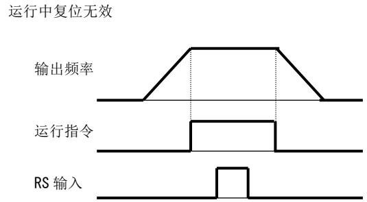
(例 4) 正常时复位无效的场合 (C102=02, 03)
