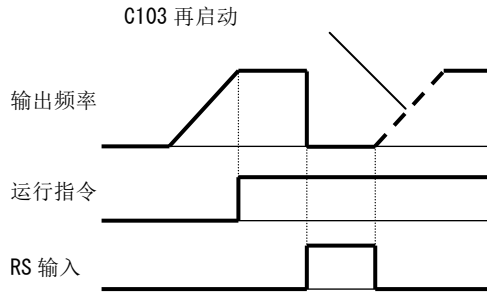
(例 3) 正常时复位有效的场合 (C102=00, 01)
