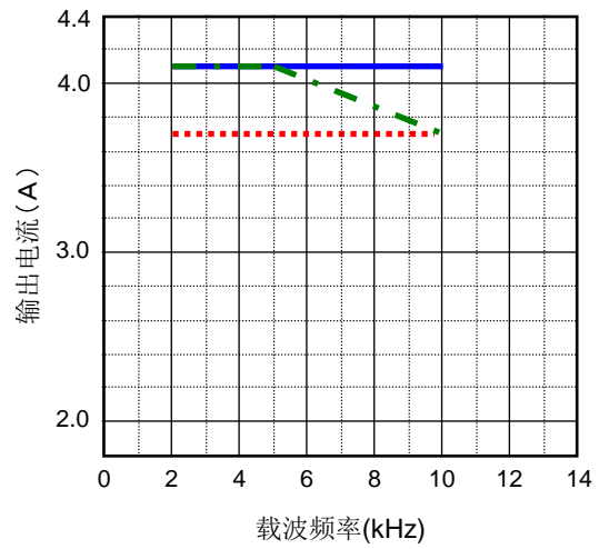
低负载规格 (4.1A)
