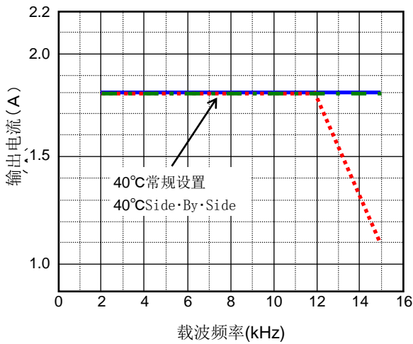
高负载规格 (1.8A)
