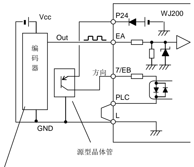
电压输出型或 PNP 集电极开路型编码器
