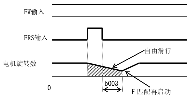
(例2) f匹配再启动 (b088=01)
