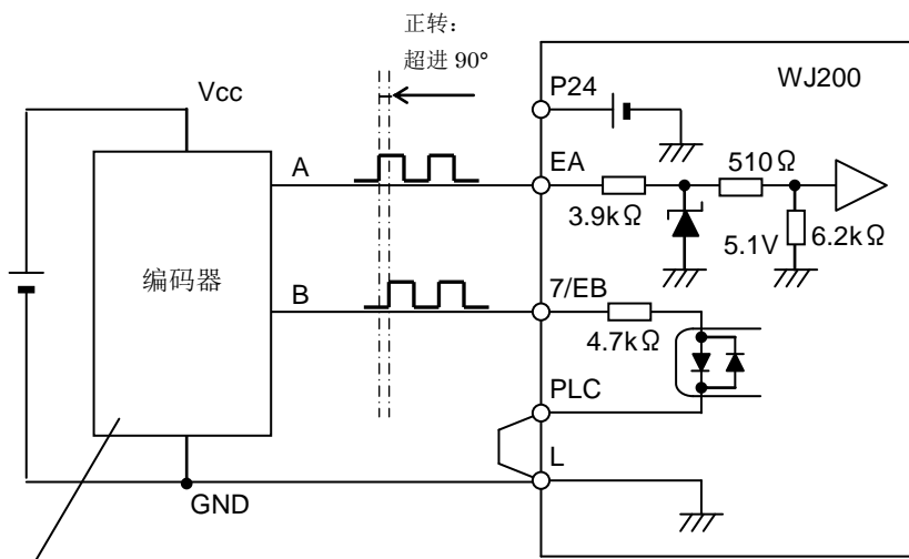
电压输出型或 PNP 集电极开路型编码器
