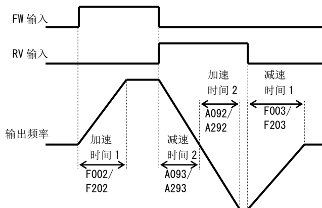
例③ 正反切换 (A094/A294=02) 的场合
