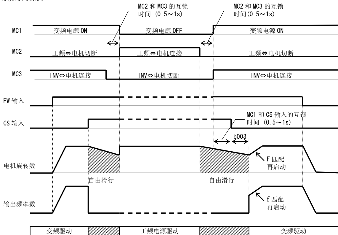
工频切换时间点例
