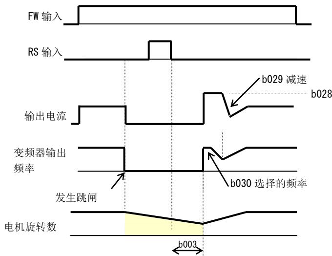
(例 6) 频率跟踪再启动
