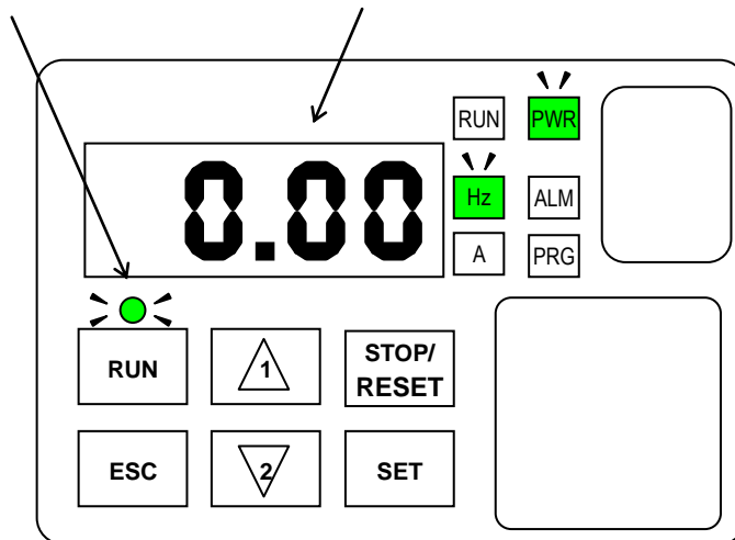
变频器启动时的显示状态
