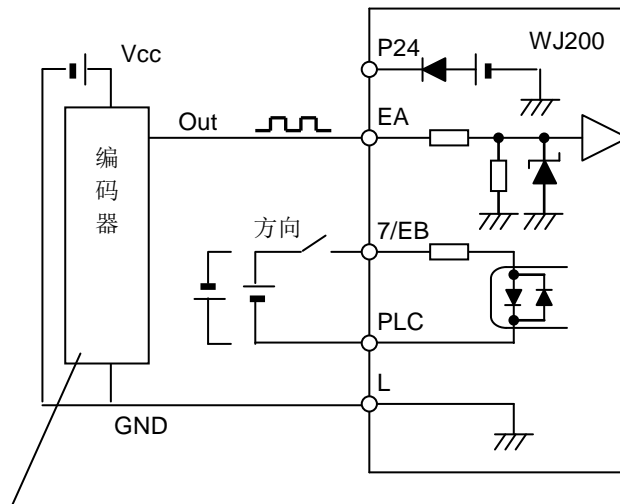
电压输出型或 PNP 集电极开路型编码器
