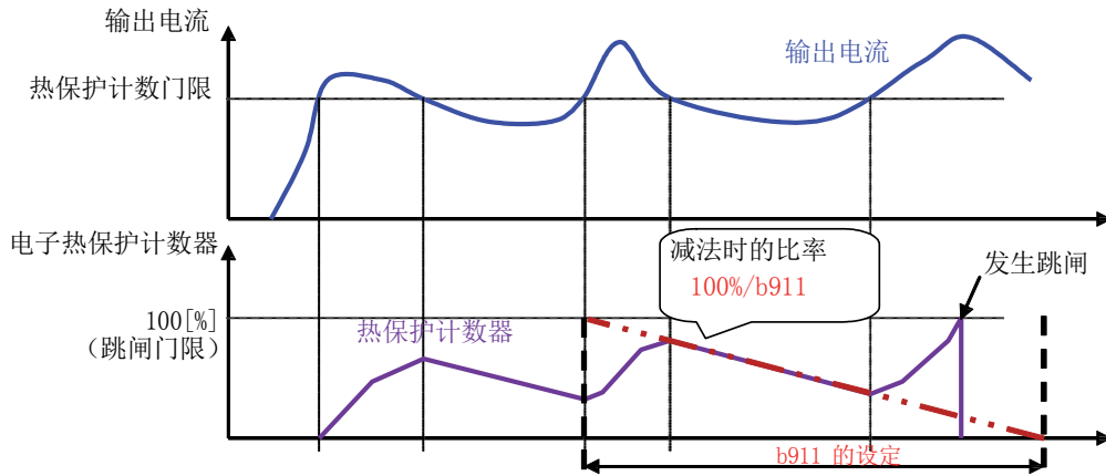
图 2. b910 = 02 时的热保护计数器减算示意图
