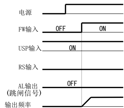
(例 3) 电源 ON 后输入运行指令 (正常动作)
