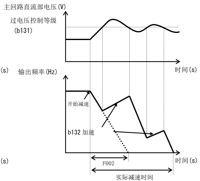
例 2) 有加速 (b130=02) 的场合
