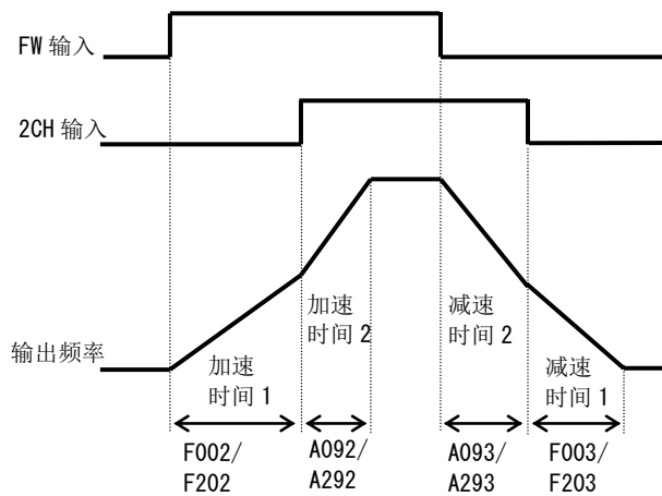
例① 输入端子切换 (A094/A294=00) 的场合
