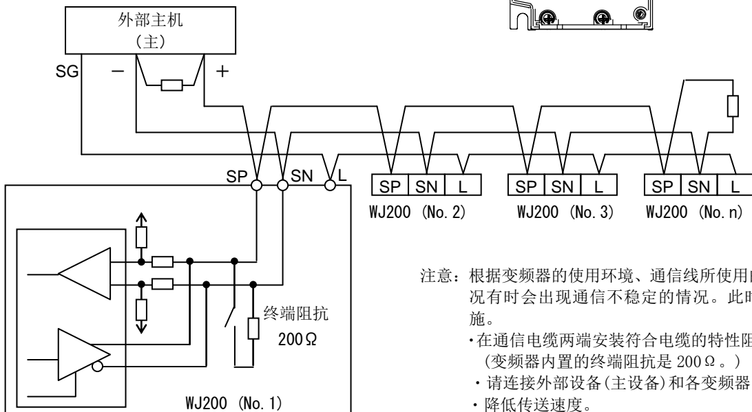
RS-485 端子
