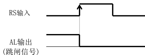
(例1)ON时跳闸解除的场合(C102=00, 02, 03)
