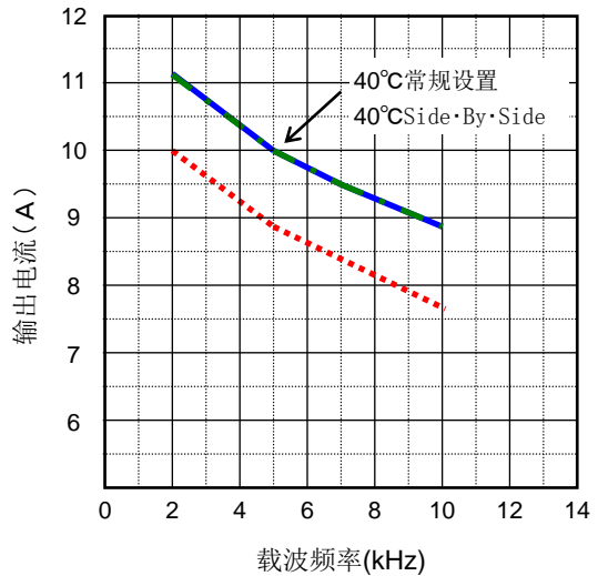
低负载规格 (11.1A)
