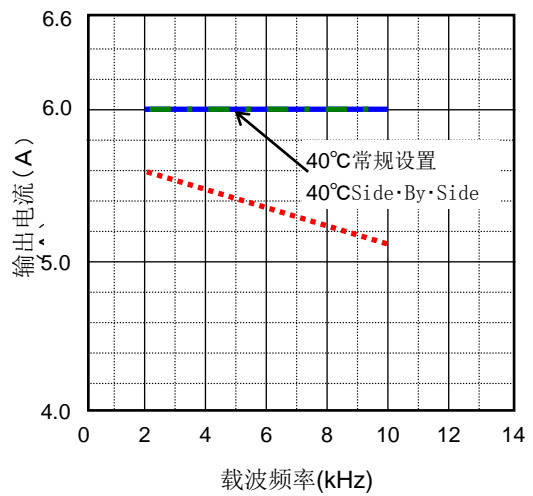
低负载规格 (6.0A)
