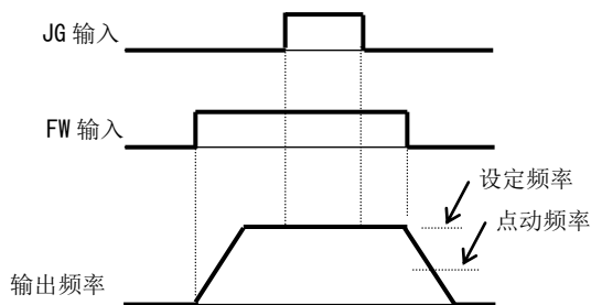
(例 1) 点动不动作的场合
