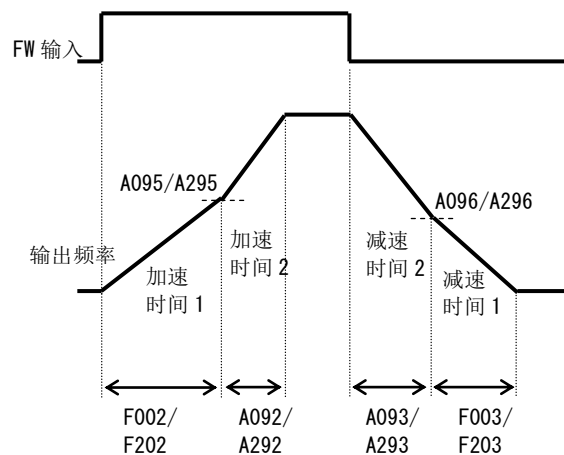
例② 频率切换 (A094/A294=01) 的场合
