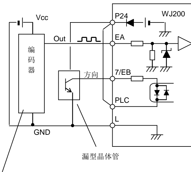
电压输出型或 PNP 集电极开路型编码器
