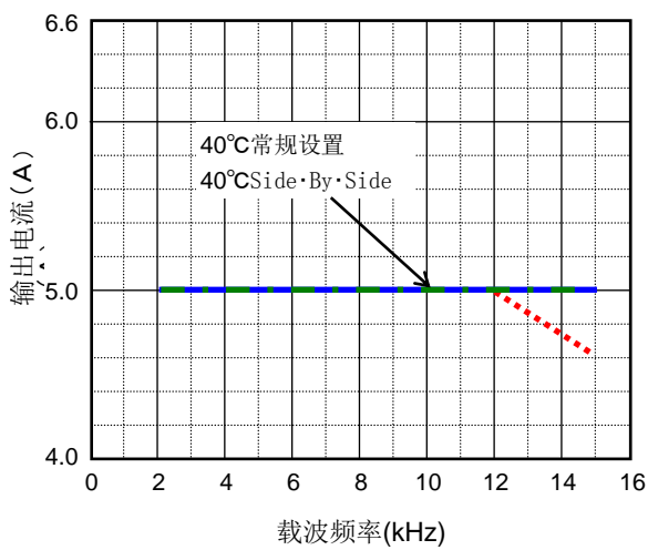
高负载规格 (5.0A)
