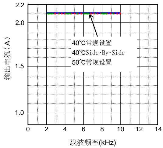
低负载规格 (2.1A)
