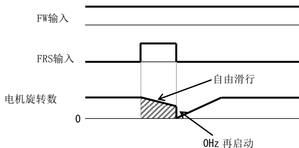
(例1) 0Hz启动 (b088=00)
