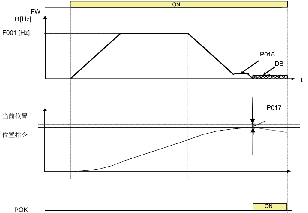
简易位置控制恢复 OFF (P080 = 0.)
