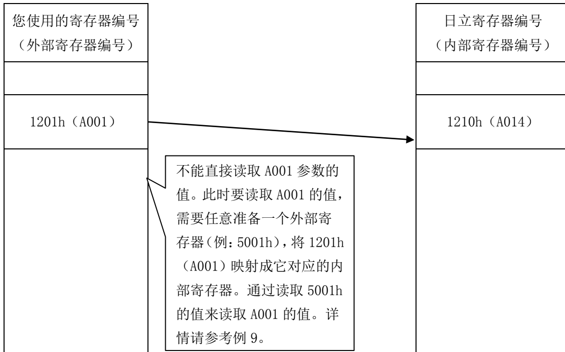
例 5 您使用的外部寄存器编号存在于日立寄存器编号 (2 寄存器长参数的高位) 一览中时
