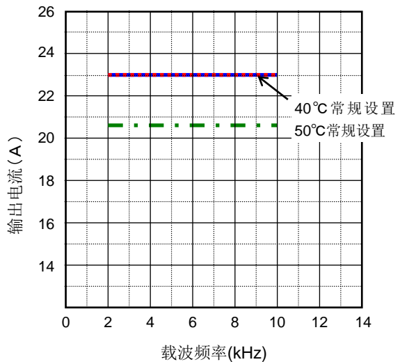
低负载规格 (23.0A)
