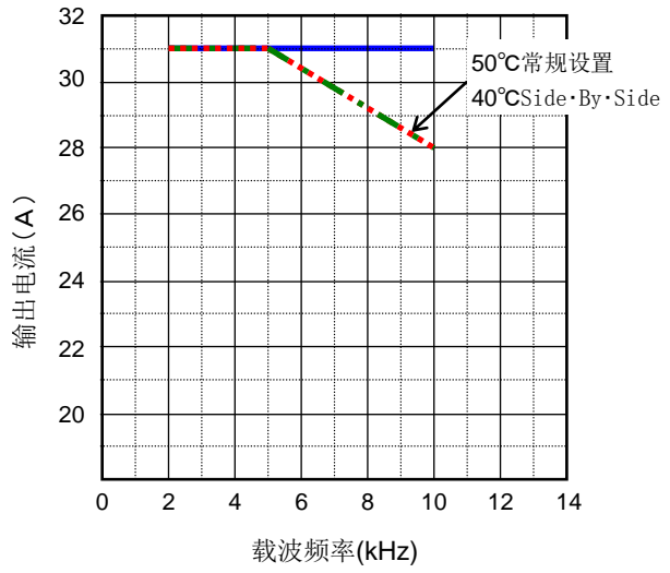
低负载规格 (31.0A)
