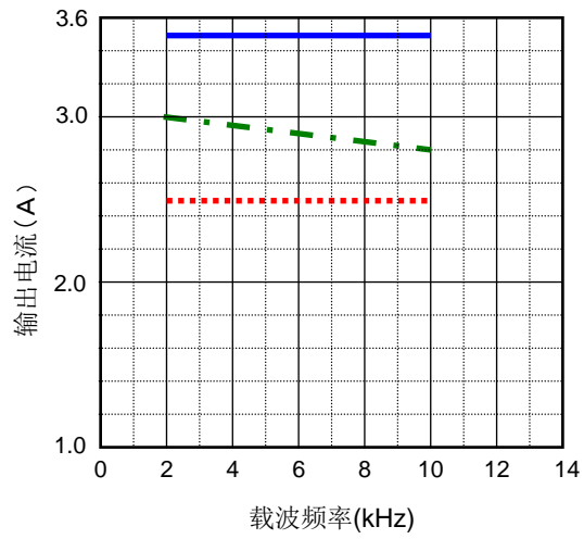
低负载规格 (3.5A)
