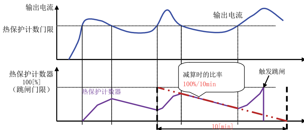
图 1. b910 = 01 时的热保护计数器减算示意图
