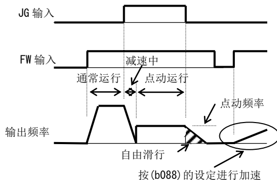
(例 2) 点动动作的场合
