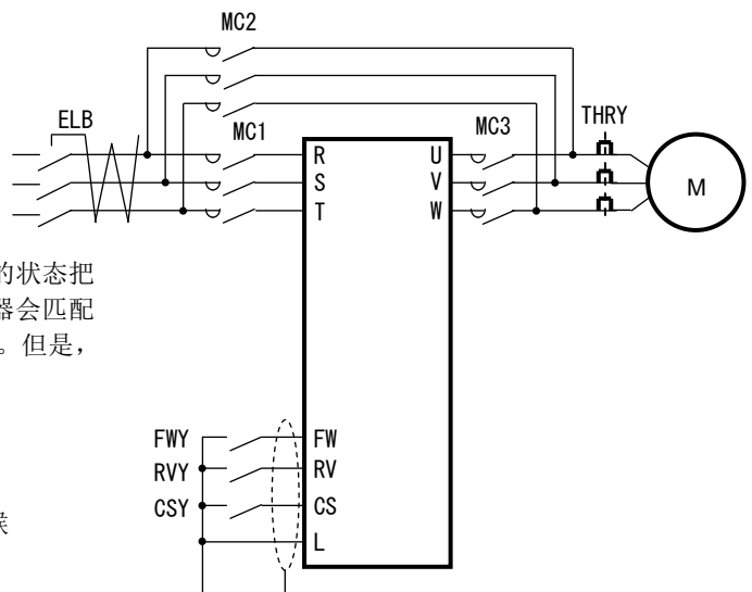
工频电源切换运行时的连接图例和时间点
