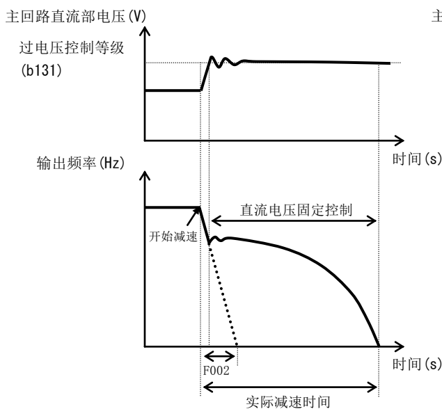
例 1) 直流电压固定控制 (b130=01) 的场合
