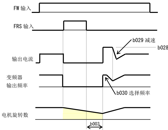
(例 3) 频率跟踪再启动 (b088=02)
