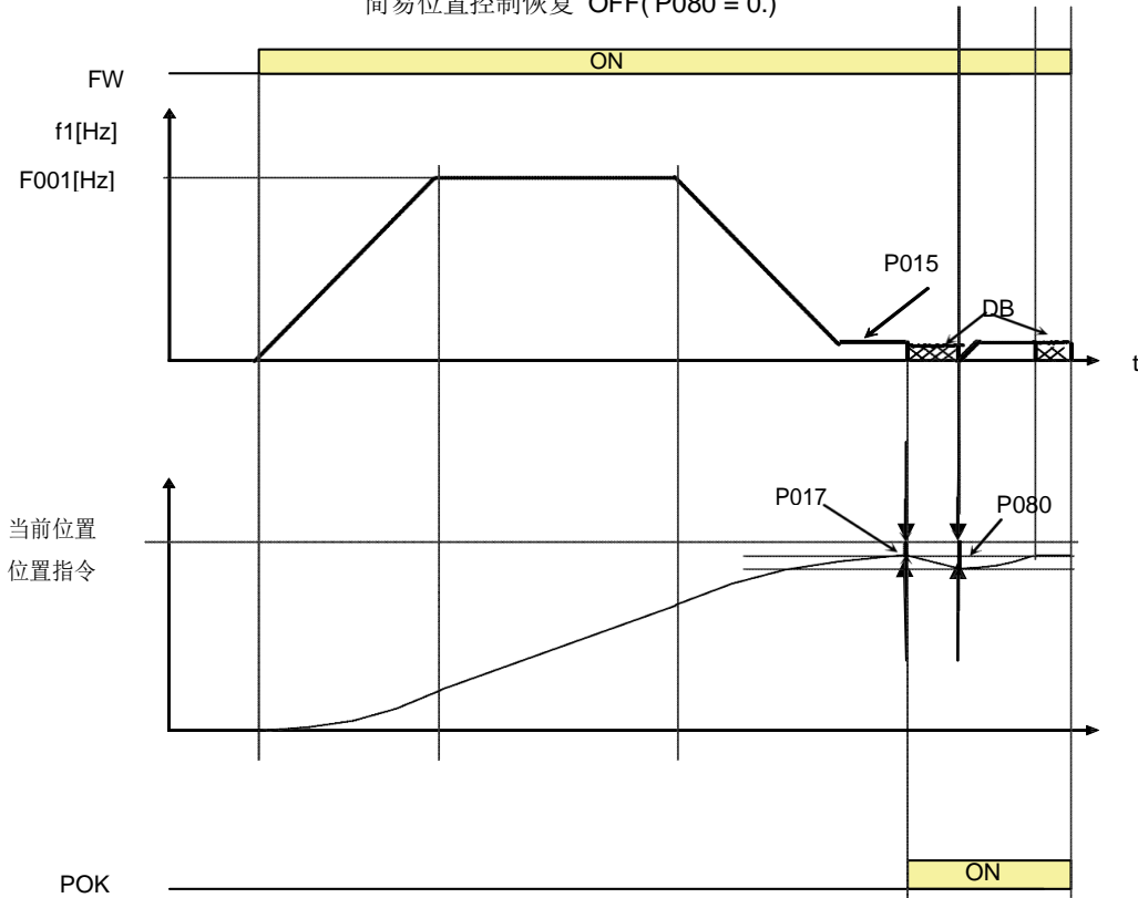
简易位置控制恢复 ON (P080 ≠ 0)
