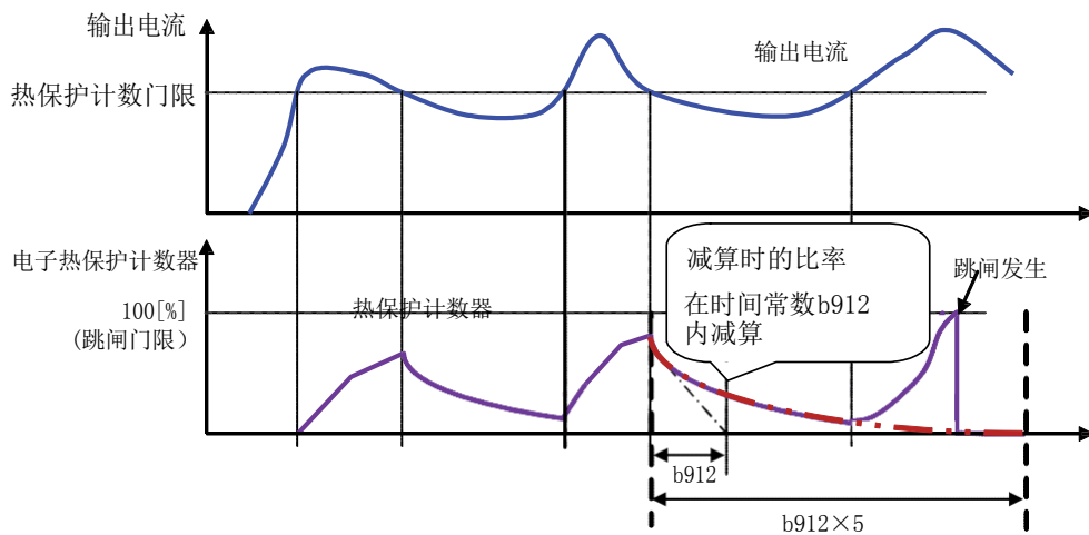
图 3. b910=03 时热保护计数器减算示意图
