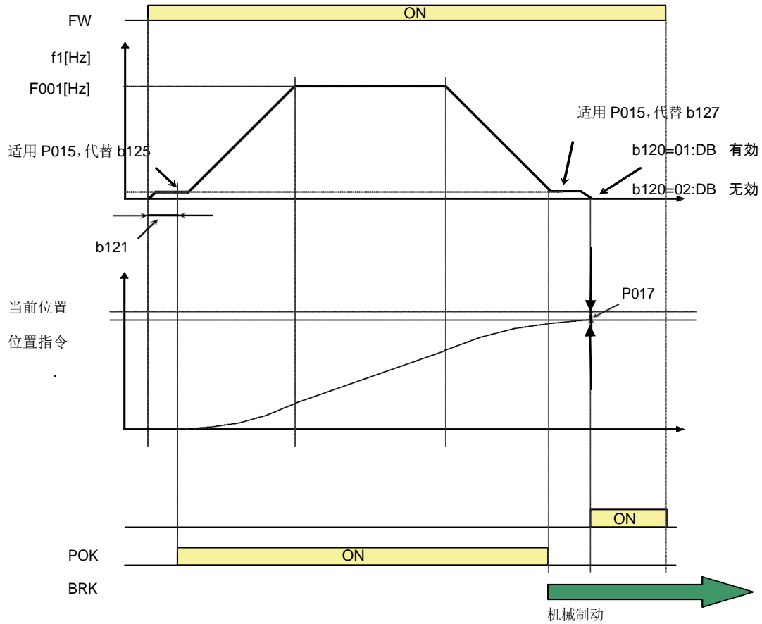
简易位置控制与制动控制功能的连动 (b120=01 or 02, P012=02)
