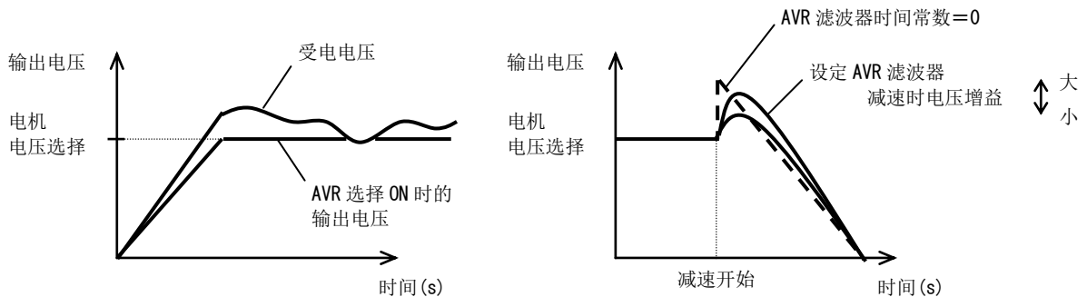
把 AVR 选择设定为减速时 OFF (A081=02) 时的例子
