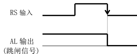
(例2)OFF时跳闸解除的场合(C102=01)
