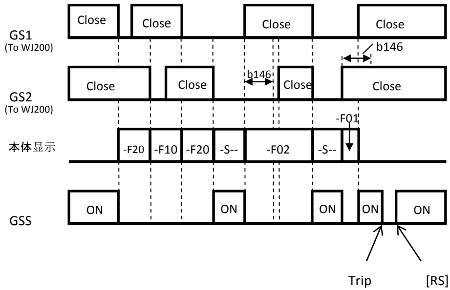
b) GSS 信号的时序图 b145=05 时
