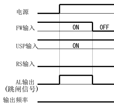
(例 1) 有运行指令时使电源 ON (运行指令 OFF 可解除)
