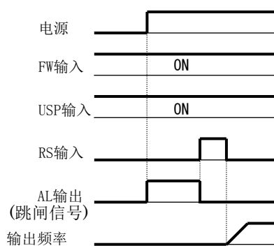
(例 2) 有运行指令时使电源 ON (复位 (RS) 可解除)
