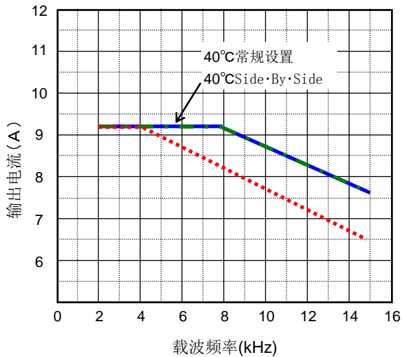
高负载规格 (9.2A)
