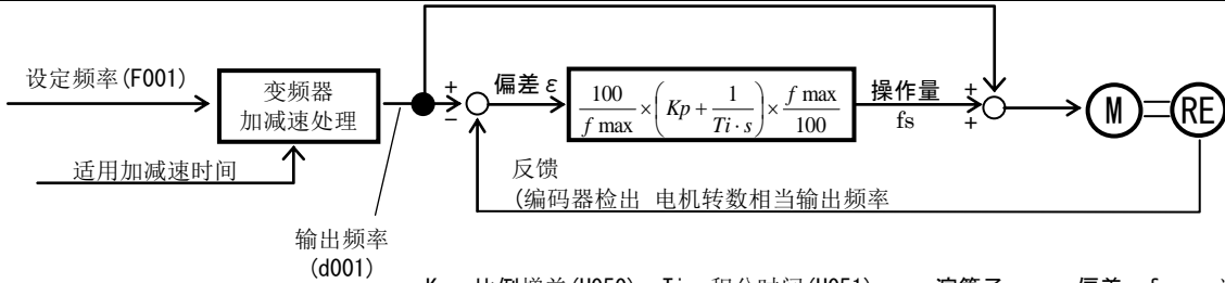
带 FB 的 V/f 控制块
