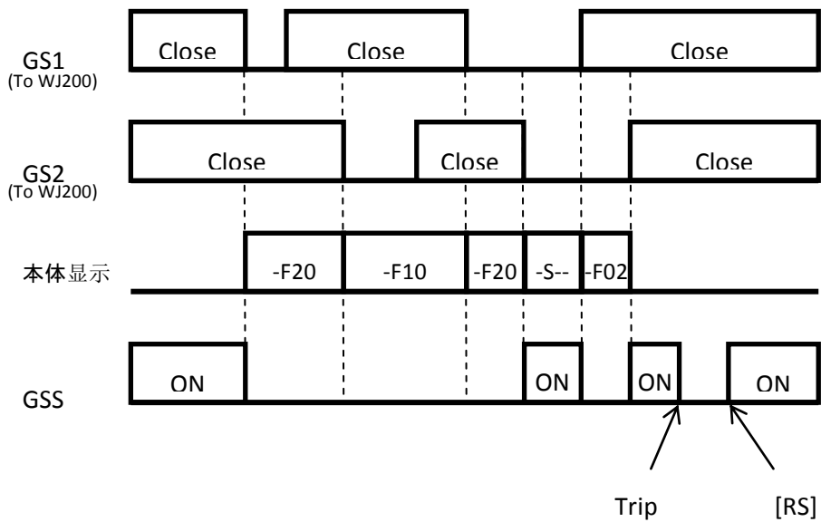
c) GSS 信号的时序图 b145=06 时
