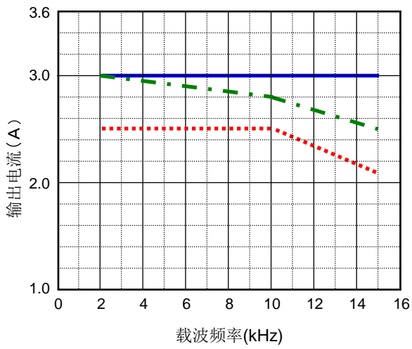
高负载规格 (3.0A)
