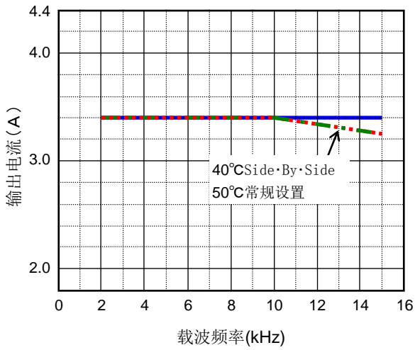
高负载规格 (3.4A)
