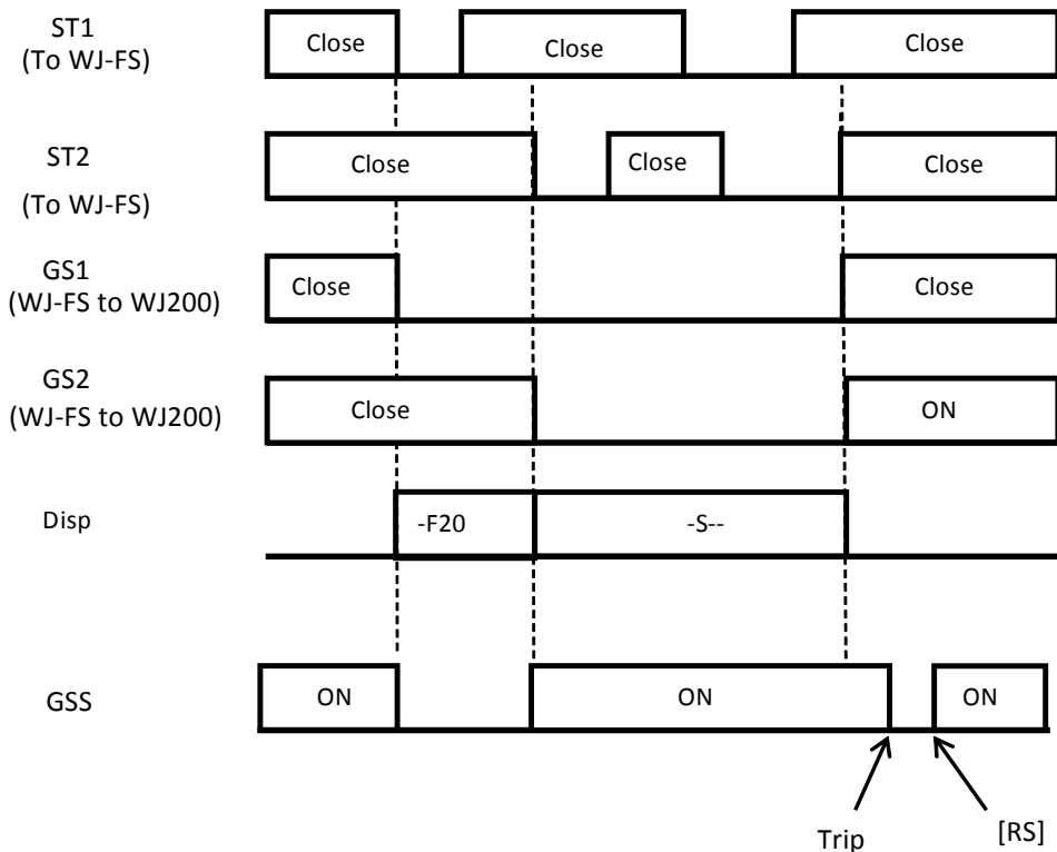
a) GSS 信号的时序图 b145=05, 06(带WJ-FS)
