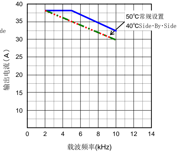
低负载规格 (38.0A)
