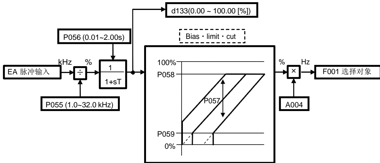
脉冲列输入框图
