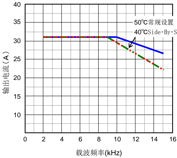
高负载规格 (31.0A)
